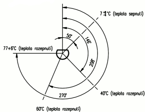
Regulační rozsah
